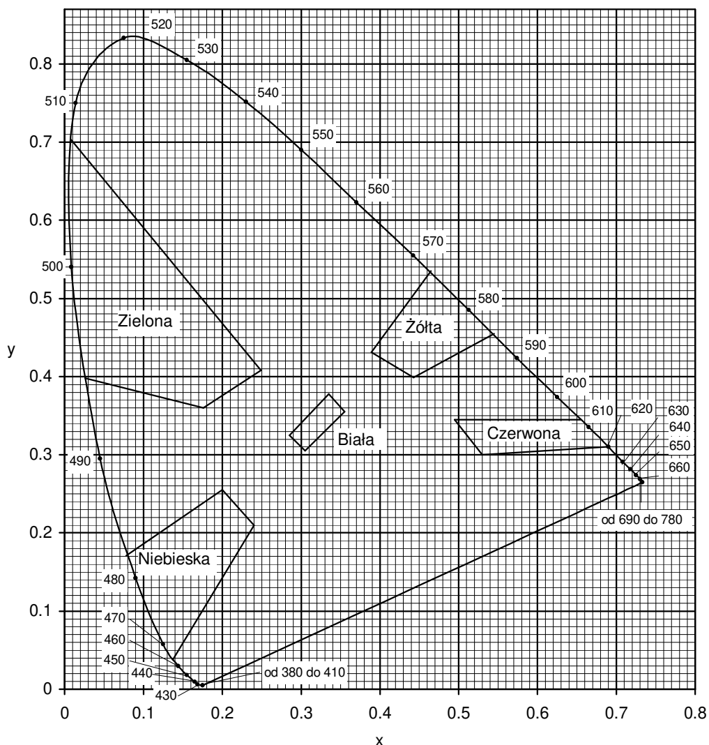
Rys. 3. Granice barw białej, żółtej, czerwonej, niebieskiej i zielonej oznakowania Pomiar współczynnika luminancji □ może być zastąpiony pomiarem współczynnika luminancji w świetle rozproszonym Qd, wg PN-EN 1436:2000 [4] lub wg POD-97 [9] i POD-2006 (po wydaniu) [10].
